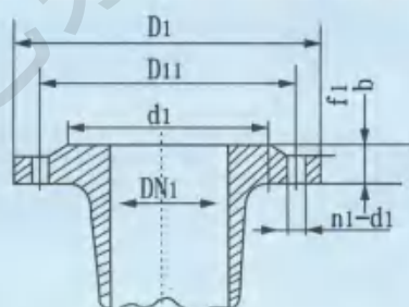
吸入口法兰
